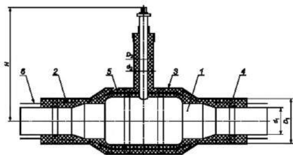
1 — шаровый кран; 2 — ППУ изоляция; 3 — защитная оболочка; 4 — центрирующая опора; 5 — электроизоляционная перфорированная трубка; 6 — проводник-индикатор СОДК (показан условно); D_1 — наружный диаметр защитной оболочки изолированного крана; D_2 — наружный диаметр защитной оболочки штока; d_1 — наружный диаметр стальной патрубка крана; d_2 — наружный диаметр штока; H — высота крана.
