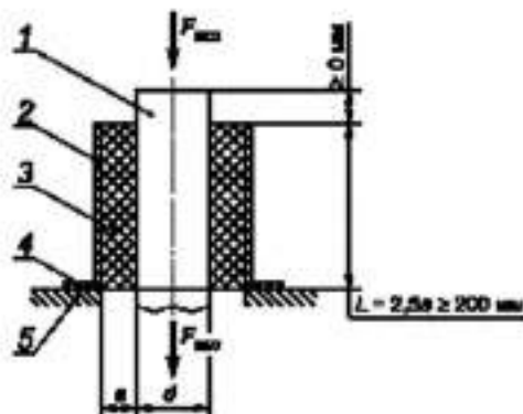
1 — стальная труба; 2 — защитная оболочка; 3 — ППУ-изоляция; 4 — направляющее кольцо; 5 — плита основания машины для испытаний; а — толщина изоляции; F_{\text{ос}} — прилагаемая нагрузка (внизу — альтернативный способ приложения нагрузки); d — см. ссылка на формулу (4).
