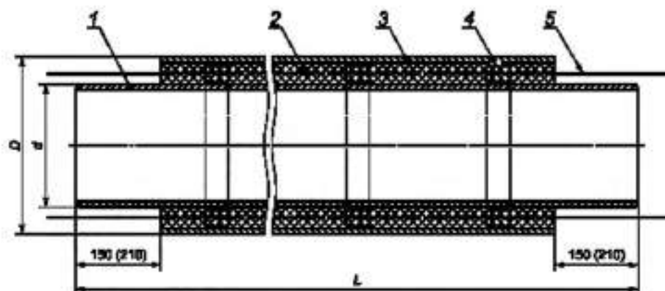
1 — стальная труба; 2 — ППУ изоляция; 3 — защитная оболочка; 4 — центрирующий опоры; 5 — проводники-индикаторы СОДК (показаны условно)
