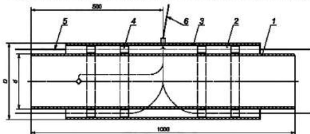
1 — стальная труба; 2 — ППУ изоляция; 3 — защитная оболочка; 4 — центрирующая опора; 5 — проводимый индикатор СОДК; 6 — кабельный вывод; D — наружный диаметр защитной оболочки; d — наружный диаметр стальной трубы
