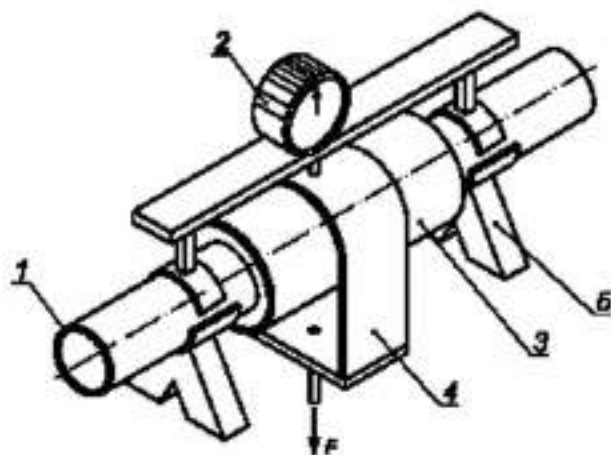
1 — стальная труба; 2 — индикатор; 3 — защитная оболочка и ППУ изолянт; 4 — приспособление для приложения нагрузки; 5 — ширина; 6 — длина; F — нагрузка
