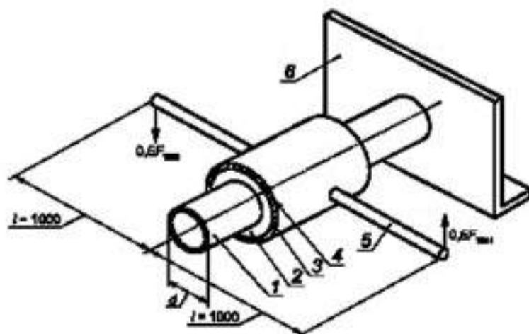
1 — стальная труба; 2 — ППУ изоляция; 3 — защитная оболочка; 4 — кожух; 5 — рычаг; 6 — неподвижная опора; F — сила; F_{\text{сдв}} — см. экспликацию к формуле (5)
