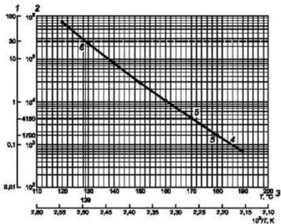
1 — ожидаемый срок службы, лет; 2 — ожидаемый срок службы; 3 — эквивалентные рабочие температуры; 4 — долговечность материала изоляции; 5 — условия ускоренных испытаний; 6 — условия эксплуатации при постоянной температуре
