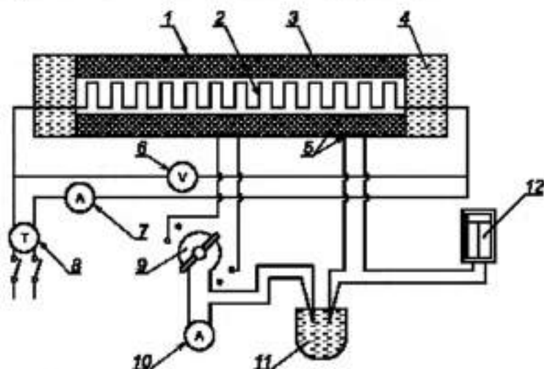
1 — стальная труба, 2 — электронагреватель, 3 — испытуемый материал, 4 — охранные секции, 5 — термометры; 6 — вольтметр, 7 — амперметр, 8 — автотрансформатор, 9 — переключатель, 10 — тальванометр, 11 — сосуд со маслом; 12 — самозаписывающий тальванометр
