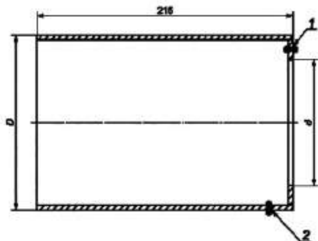
1 — герметизатор кабельного вывода, 2 — закрывное отверстие, D — наружный диаметр заглушки, d — диаметр монтажного отверстия заглушки (под сварку)
